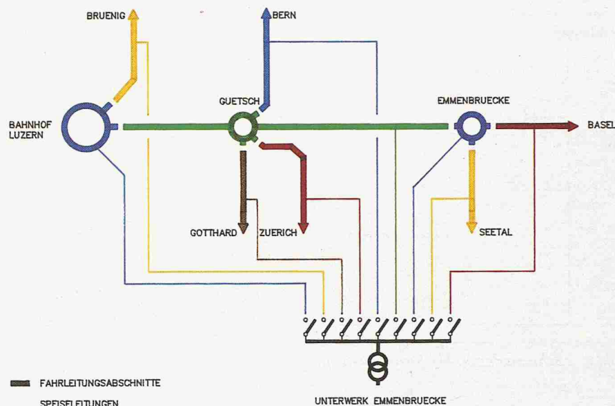
Bild 1. Speiseabschnitte der Fahrleitungen der Region Luzern
