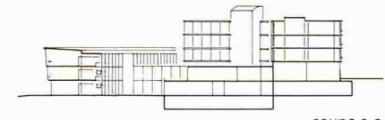
coupe c-c
