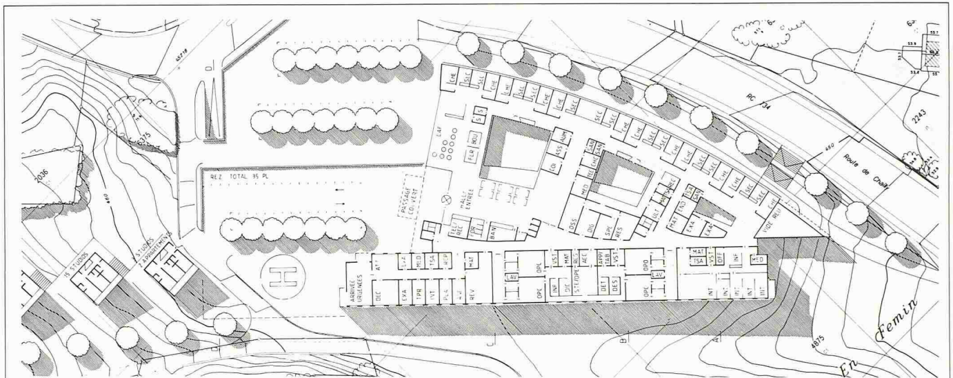
rez-de-chaussée 1:1500
