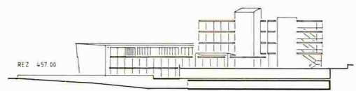
coupe d-d
