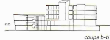
coupe b-b
