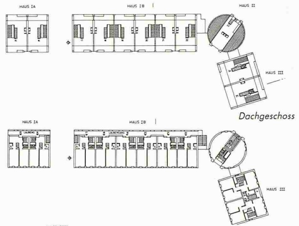
2. Obergeschoss
