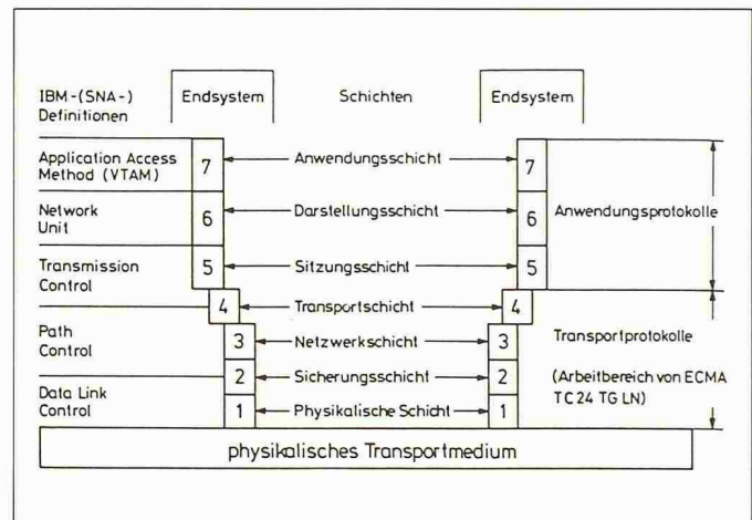
Bild 5. Das ISO/OSI-Modell
