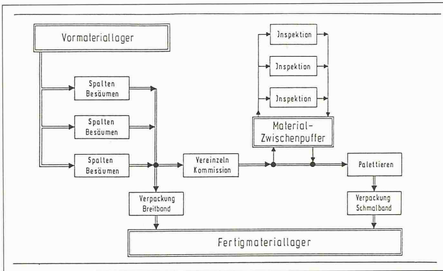
Bild 1. Strukturbild der Elektroband-Zurichtung. In der automatischen Zurichtung für Elektroband wird durchlaufgeglühtes bzw. isoliertes Breitband in den Stufen – Besäumen/Spalten – Vereinzeln – Zwischenpuffern/Sanieren – Palettieren – Verpacken – zu versandfähigem Schmalband verarbeitet. Zur logistischen Entkopplung des Sanierens (Nacharbeiten) ist ein zusätzlicher Materialpuffer installiert
