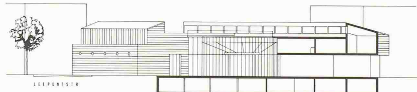
Schnitt Fussgängerpassage
