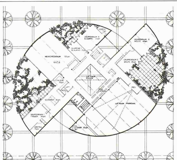
1. Obergeschoss
