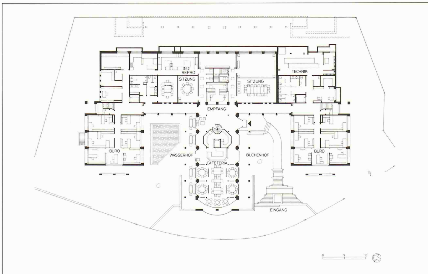
Bild 12. Grundriss Eingangsgeschoss
