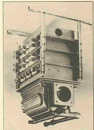
Bild 2. Bomat-Heizkesselkörper ohne Isolation und Verschalung
