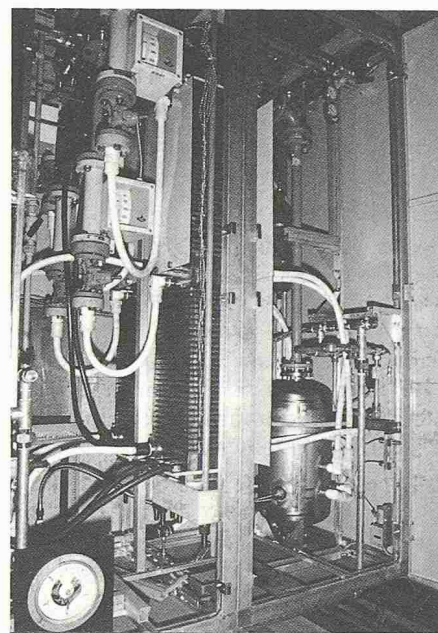
Bild 2. Versuchsaufbau mit 4 MEMBREL – Zellblöcken à 5 Nm 3 /h, Quelle: ABB Zürich
