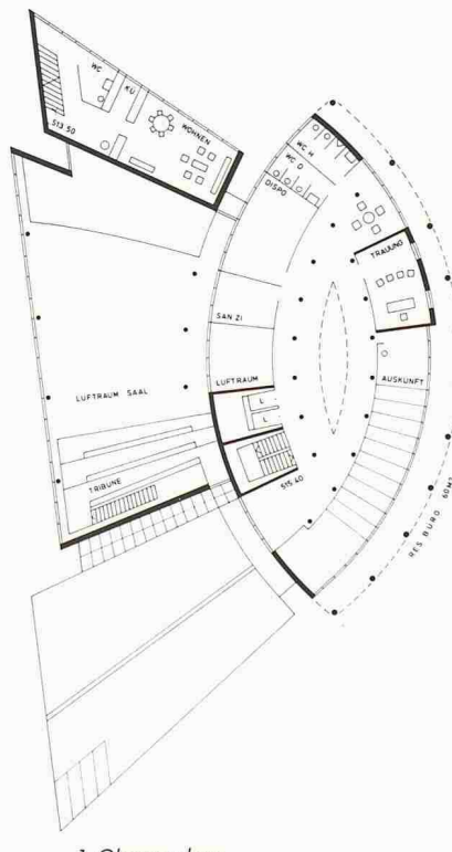
1. Obergeschoss
