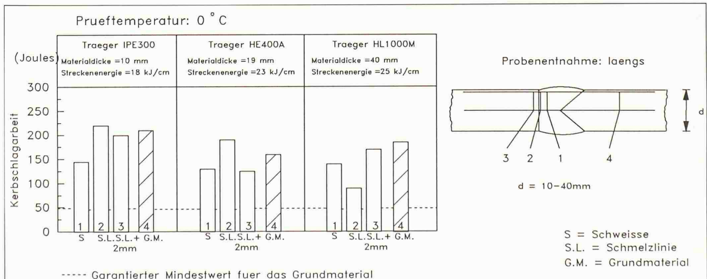
Bild 5. Charpy V-Kerbschlagbiegeversuch auf einer Lichtbogen-handgeschweissten Schweißverbindung
