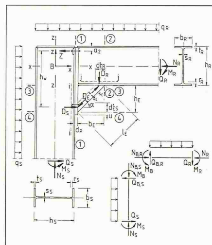
Bild 14. Berechnungsmodell für geschraubte Verbindungen
