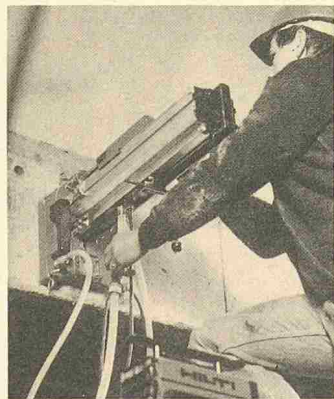
Diamantbohrgerät DCM1
