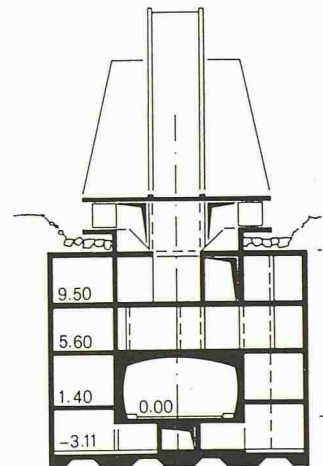
Coupe A-A
