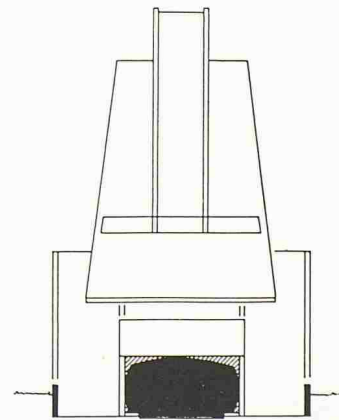
Vue frontale
