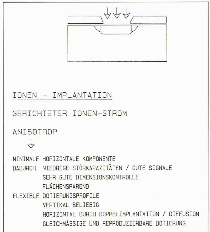
Bild 18. Technologieentwicklung der Dotierungs- und Heissprozesse
