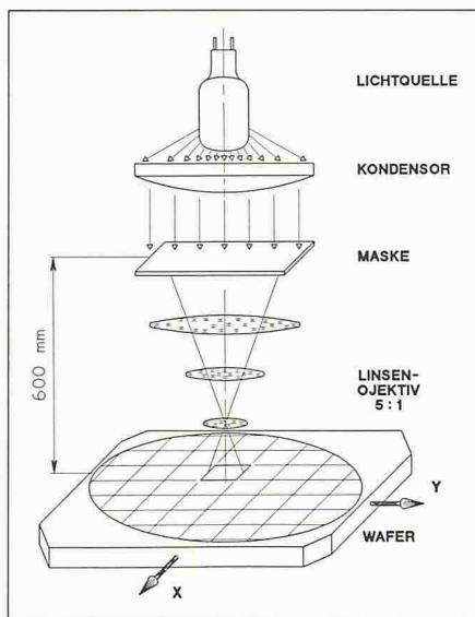
Bild 17. Step- und Repeat-Belichtungsprinzip
