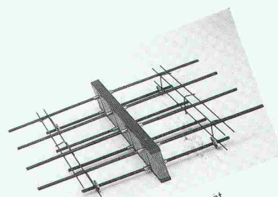
Kragplatten-Anschluss Standard-Element
