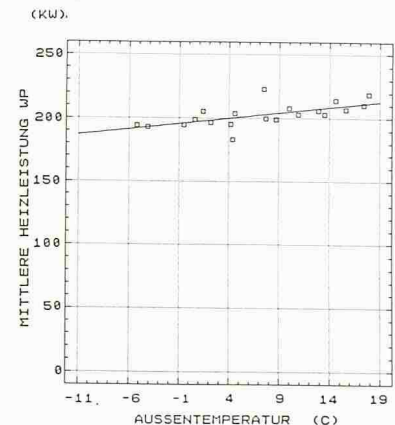
Heizleistung der Wärmepumpe, Messdaten 1984-1986
