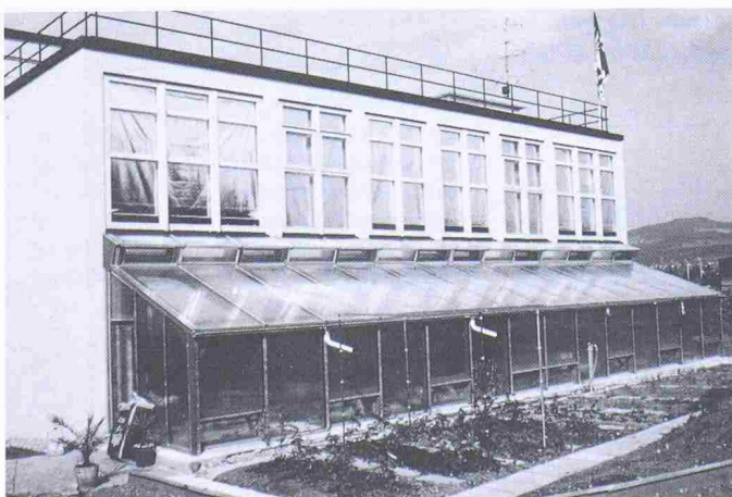
Bild 7. Südostfassade mit Gewächshaus im EG und Luftkollektoren im OG, Stellung Sommerbetrieb, d.h. die Luftabsorber sind mit reflektierenden Rollos abgedeckt
