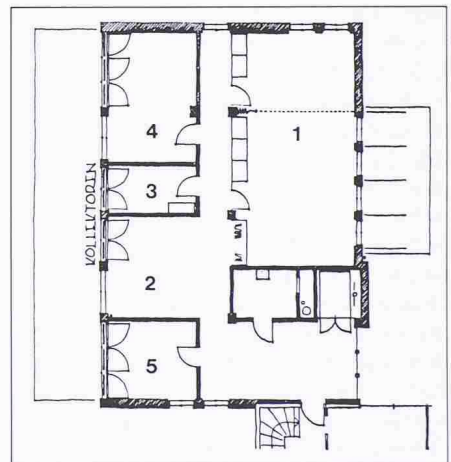
Bild 2. Grundriss Obergeschoss; 1 Besprechung, 2 Ausstellung, 3 Labor, 4 Reparaterraum, 5 Messraum
