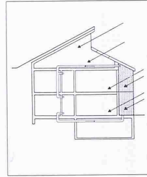
Verglaste Veranda: Die zweigeschossige Veranda ist eine unbeheizte Wohnraumerweiterung. Als solche vermindert sie die Wärmeverluste der grosszügig verglasten Wohnzone (Pufferaum). An sonnigen Wintertagen soll sie zudem Warmluft in die Nordzone liefern
