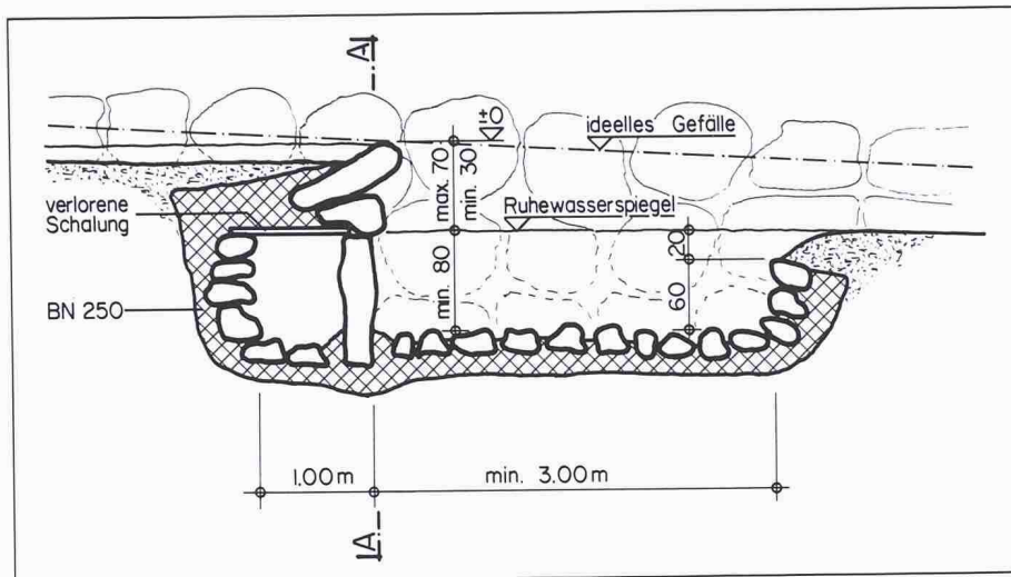
Bild 3. Fischbecken, Längsschnitt
