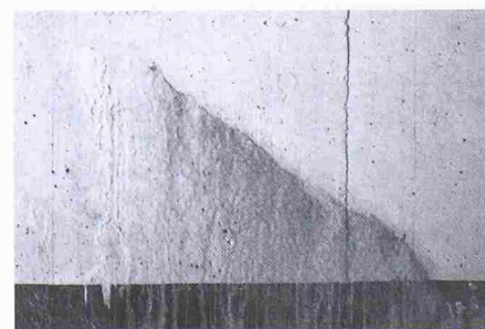
Bild 3. Aussinterungen bei einem wasserführenden Trennrisse
