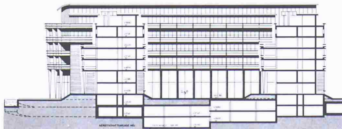
Schnitt B-B
