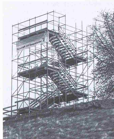
Die Interessengemeinschaft SiGe Zug erstellte auf der Zuger Guggiwiese einen 10 m hohen Aussichtsturm, der der Öffentlichkeit bis Ende Mai frei zugänglich ist. Mit ihm soll demonstriert werden, dass ein fachgerecht erstelltes Baugerüst Unfälle wirksam verhüten kann (Bild Z. Ruepp)
