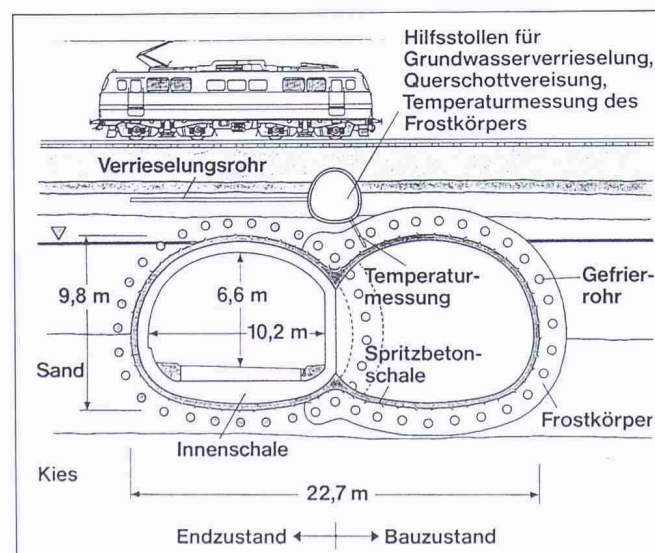
Bild 5. Fahrlichtunnel Mannheim im Schutze eines Tragringes aus gefrorenem Boden bergmännisch in Spritzbetonbauweise aufgeföhrt (Querschnitt links, Längsschnitt rechts) (Dusch/Mayer)
