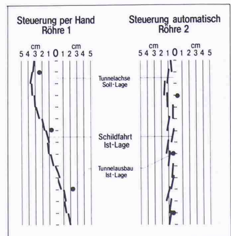
Bild 2. Verbesserung der Hydro-Schildführung beim Auffahren des Tunnels Viljejust/Frankreich durch automatisch gesteuerten Betrieb (Babendererde)
