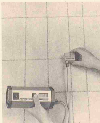
Bewehrungssucher Profometer 3
