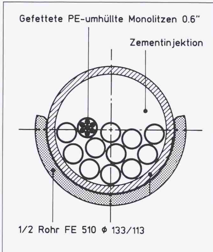
Bild 4. Spannkabel auf einem Umlenksattel bei einem Zwischenaufleger
