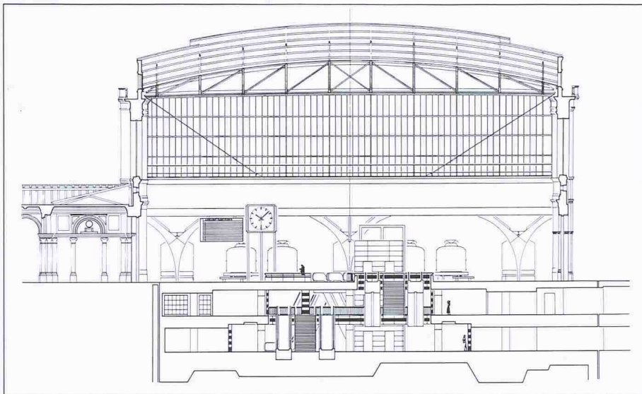
Bild 10. Querschnitt Haupthalle
