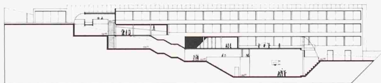
fa  ade nord-ouest
