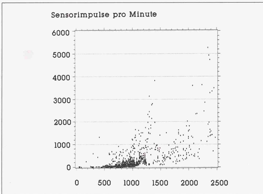
Bild 4. Der Streubereich der Impulzzahlen bei gegebenem Reinwasserabfluss ist enorm gross. Anhand diese Beispiels (Zusammenfassung der Daten von 4 Ereignissen aus dem Sommer 1990) wird dies deutlich. Man erkennt, dass beispielsweise bei einem Abfluss von etwa 2,4 \text{ m}^3/\text{s} während einer Minute etwa 750 Impulse, während einer anderen 5300 Impulse registriert wurden.
