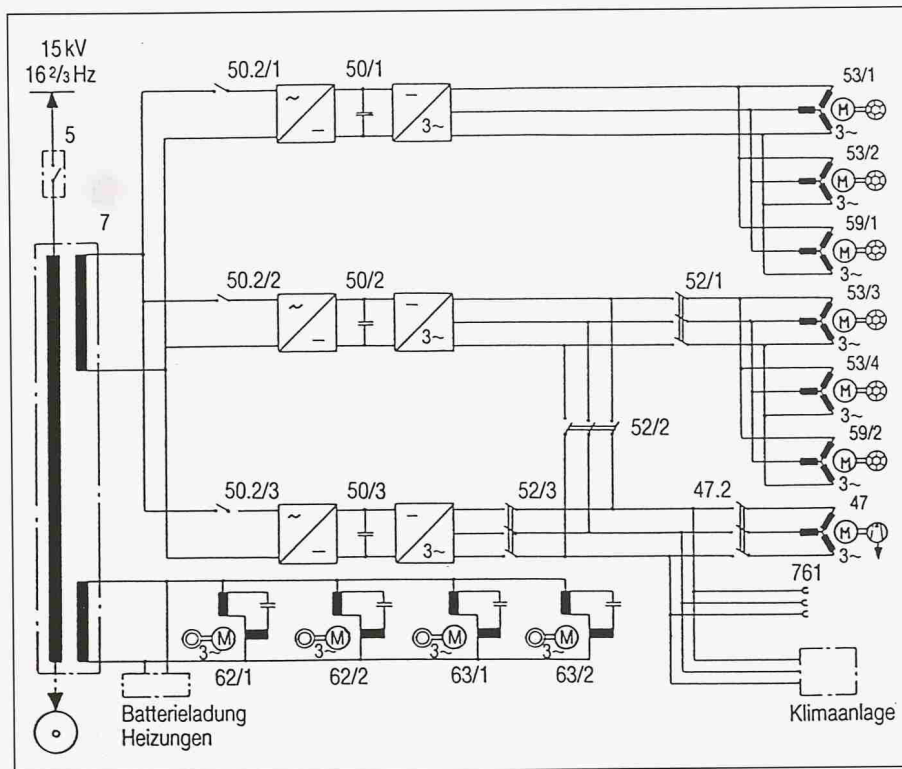
Bild 5. Prinzipschema der Hilfsbetriebe der Re 4/4 450. Es bedeuten: 5 Hauptschalter, 7 Transformator, 47 Kompressor, 47.2 Schütz für Kompressor, 50 Bordnetzumschalter (BUR), 50.2 Schütz für BUR, 52 Schütz für Kompressor-Umschaltung (BUR-Wechsel), 53 Lüftermotor für Fahrmotorkühlung, 59 Lüftermotor für Ölkühlung, 62 Transformator-Ölpumpe, 63 Umrichter-Ölpumpe und 761 Kupplungsdose für Speisung der Klimaanlage im Steuerwagen (Zeichnung SBB)
