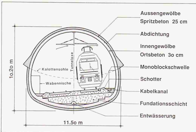
Bild 3. Tunnelnormalprofil
