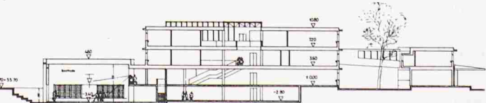
Querschnitt Sporthalle
