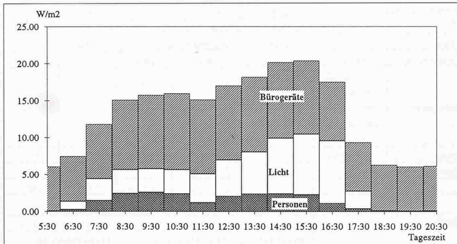
Bild 6. Typischer Tagesgang der internen Lasten für das Bürogebäude Nixdorf während der Wintermessung
