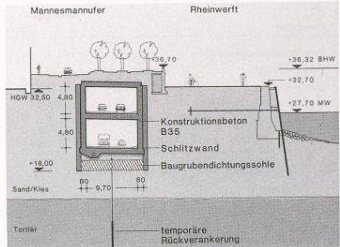
Bild 5. Rheinufertunnel in Düsseldorf
