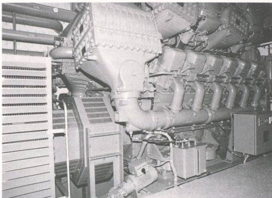
Bild 3. Deselektische Notstromanlage; Leistung 4500 kVA
