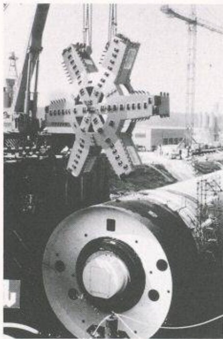
Bild 15. Erstellung des Grauholtzunnels bei Bern in Schildbauweise. a) Einsetzen des Schneirades; b) Geologie
