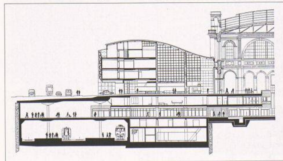
Bild 7. Querschnitt durch den neuen Nordtrakt. Links S-Bahn-Kasten, rechts Hallenausbaue
