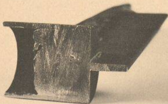
Schnitt durch die Cadweld-Schweissung. Band und Kabel sind molekular fest verbunden.
