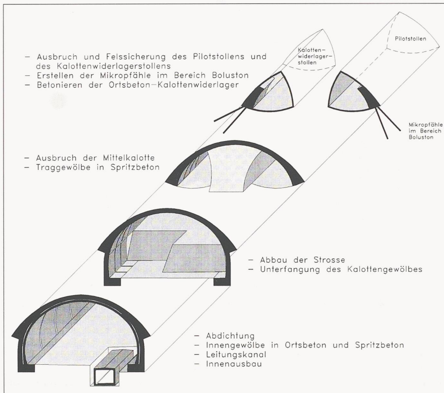
Bild 5. Bauvorgang Verzweigung
