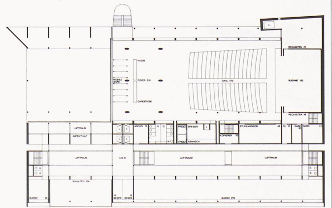
1. Obergeschoss
