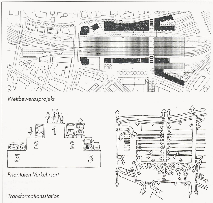
Bild 3. Gesamtüberbauung
