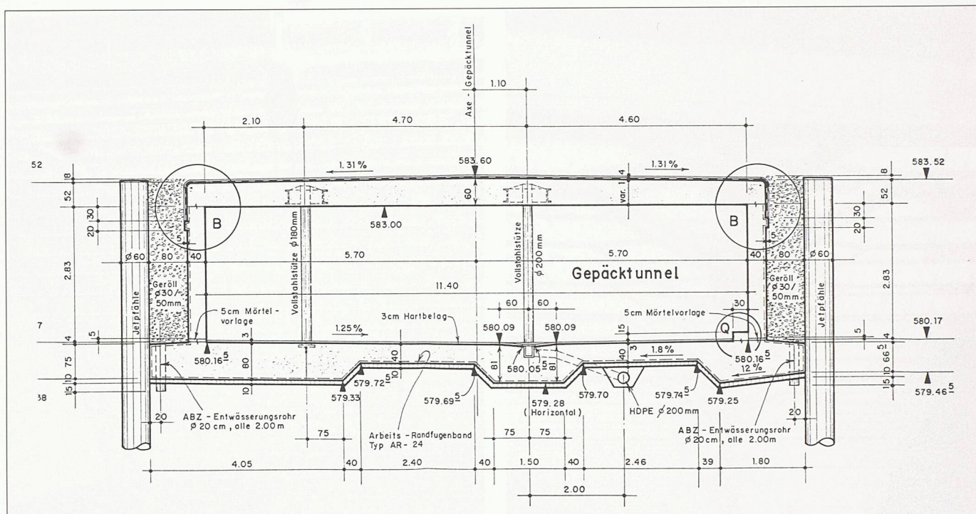
Bild 8. Gepäcktunnel PTT
