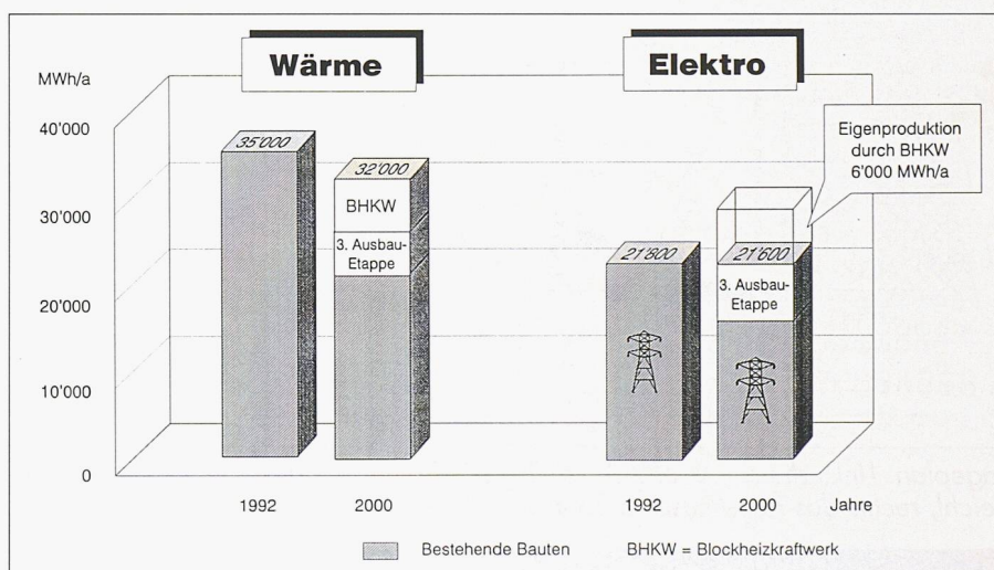
Bild 6. Energiebilanzen ETH Hönggerberg 1992/2000, nach Ausbau der 3. Etappe und unter Berücksichtigung der Sanierungsmassnahmen
