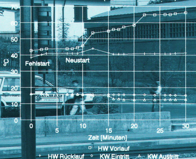
Anfahrversuch GMWP (kleine Drehzahl, Kaltstart)
