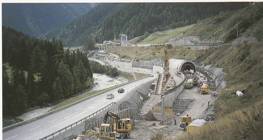
Bild 9. Baustelle Klosters-Selfranga
