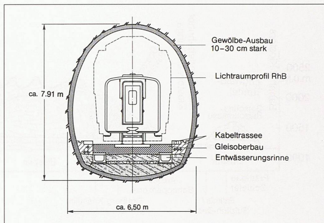
Bild 5b. Konventionell vorgetriebener 1-Spur-Tunnel
