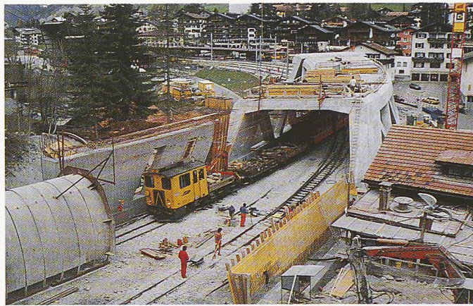
Bild 11. Fertigstellung der neuen Gleise nach dem Einschleichen der Brücke im April 1993
