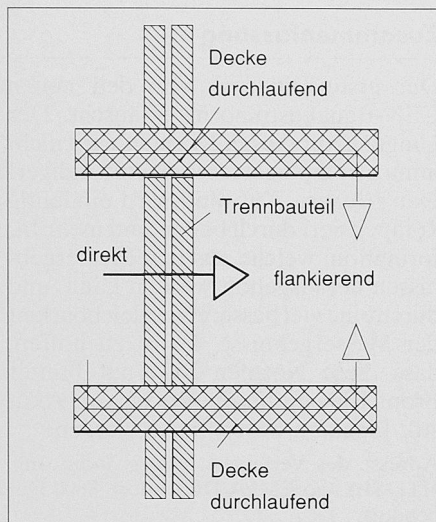
Bild 1. Zweischalige Trennbauweise mit durchlaufender Decke
