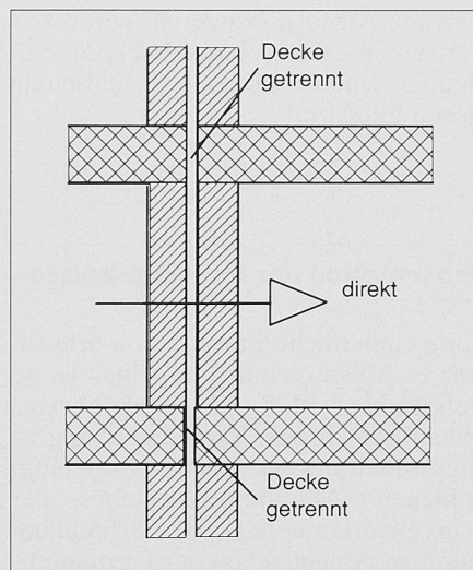
Bild 2. Zweischalige Trennbauweise mit getrennter Decke
