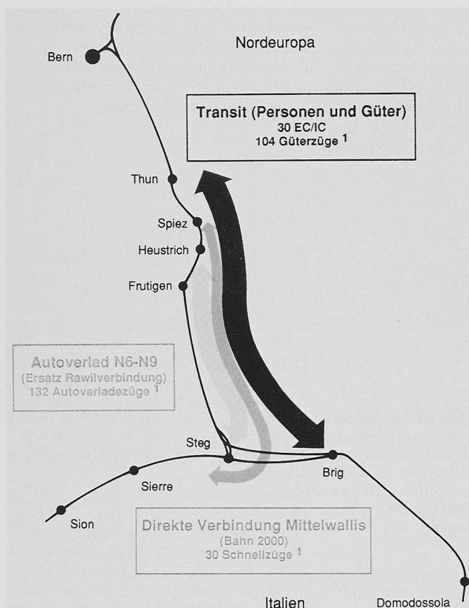
Bild 2. Die drei Funktionen der Lötschberg-Basislinie (Kapazität der Linie, Anzahl Züge pro Tag in beiden Richtungen zusammen)
