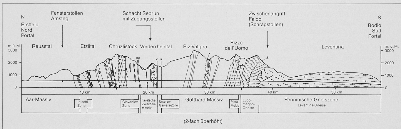
Bild 1. Geologisches Längenprofil des 57 km langen Gotthard-Basistunnels. Zwischenangriffe erfolgen in Amsteg UR, Sigrun GR und Faido TI
