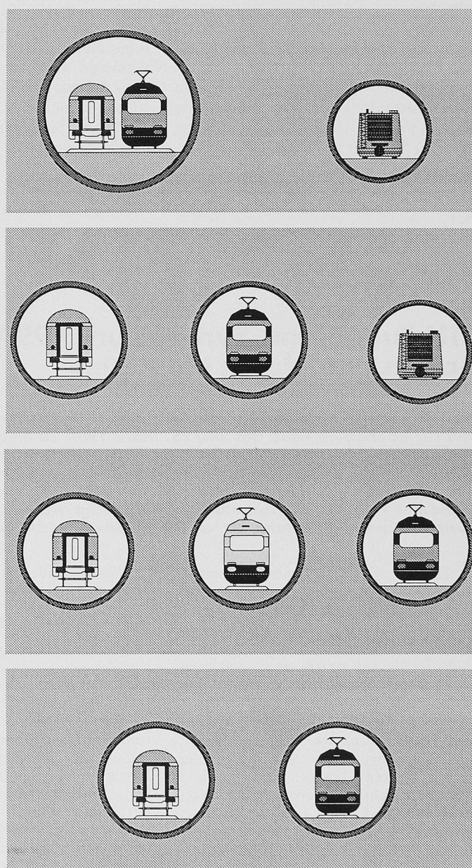
Bild 4. Tunnelsystemvarianten. Für den Gotthard-Basistunnel ist die Wahl auf zwei parallele Einspurrohre (unterste Variante) mit regelmässigen Querverbindungen und Möglichkeiten zum Gleiswechsel (Bild: Basler & Partner AG)
