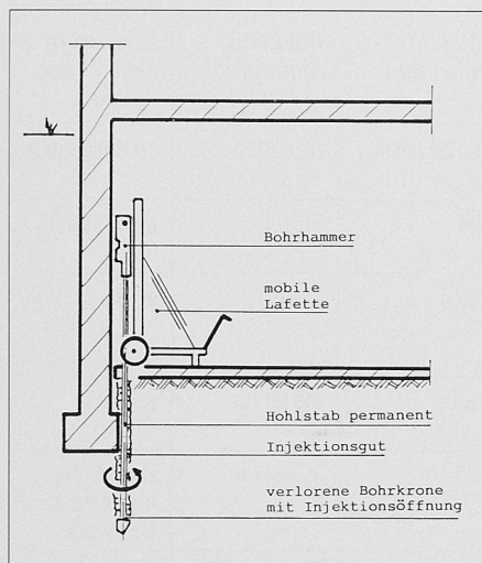
Bild 3. Injektionsbohrpfahl
