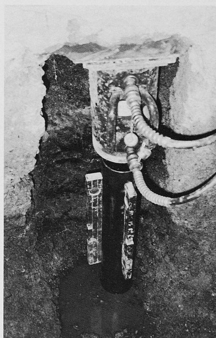
Bild 7. Presspfähle, Objekt Birmensdorferstr. 326, Zürich (alle Bilder: Ter-ratech AG)
