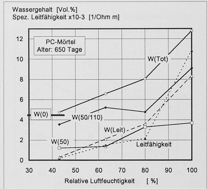
Bild 4. Der bei 50 °C, zwischen 50 und 110 °C und der totale, bei 110 °C verdampfbarer Wassergehalt ( W_{50} , W_{50/110} und W_{Tot} , ausgezogene Linien) und der elektrisch leitfähige Wassergehalt W_{Leit} (gestrichelte Linie) sowie die spezifische elektrische Leitfähigkeit (punktirierte Linie) des PC-Mörtels als Funktion der Auslagerungsfeuchtigkeit. Eingetragen ist auch der elektrisch nichtleitende Wassergehalt W^0
