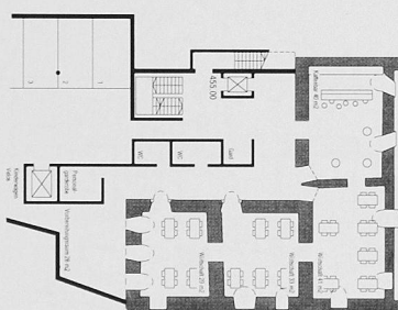
1. Untergeschoss
