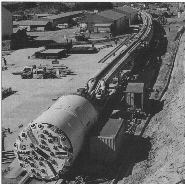
Teleskopschildmaschine TB 539 H/MS für 5,39 m \emptyset , Lesotho
