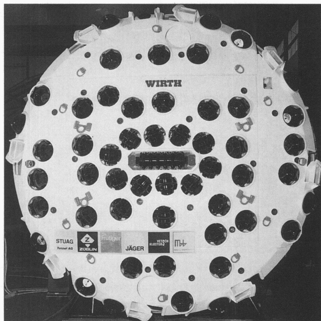
Bohrkopf der TBE 770/850, für 7,69 m \emptyset , Vereina
