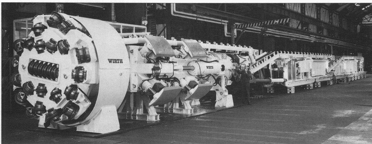
Vollschnitt-Tunnelbohrmaschine TB 350 E für 3,5 m \emptyset , Korea
