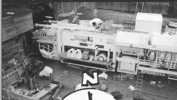
Konsolidierungsbereich am Nordportal des Vereinatunnels
