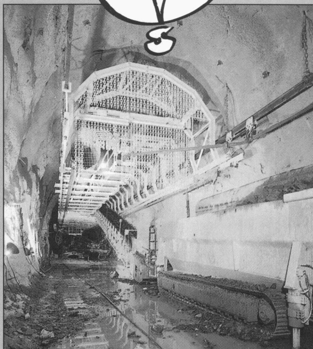
Hängebühne für den konventionellen Vortrieb in der Einspurstrecke Vereinatunnel Süd
