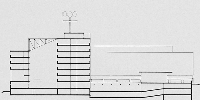
Schnitt Nord-Süd
